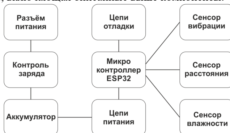
Рисунок 5– Функциональная схема модуля датчиков
