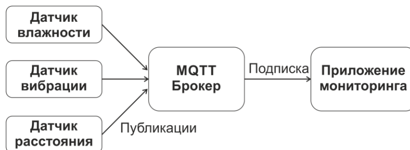
Рисунок 4 - Схема передачи данных с использованием протокола MQTT
